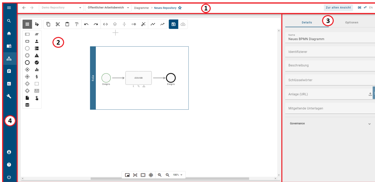
Abbildung: Die Designer Oberfläche unterteilt sich in Explorer (1), Arbeitsbereich (2), Details und Optionen (3), und Menüleiste (4).
